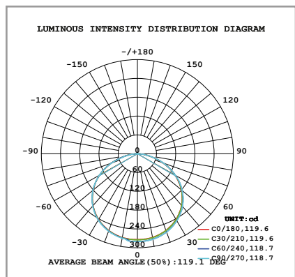
Fotometria - Eficacia: 100 lm/w
